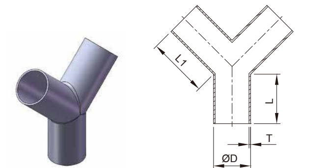
28W 90° Y TRUE WELD END
