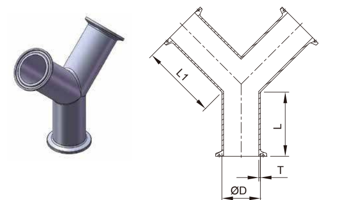
28BMP 90° Y TRUE CLAMP END
