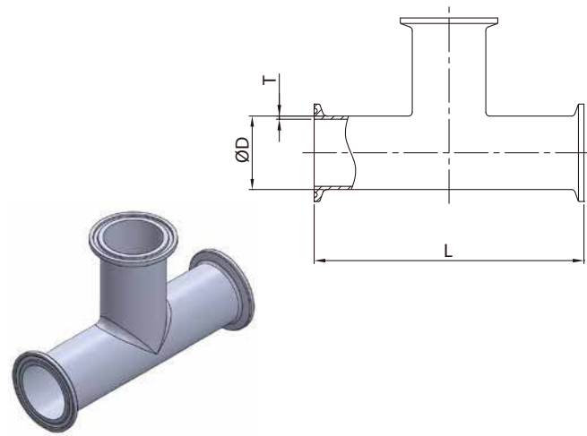
DT-4.1.2-4T CLAMP TEE (DT-18)
